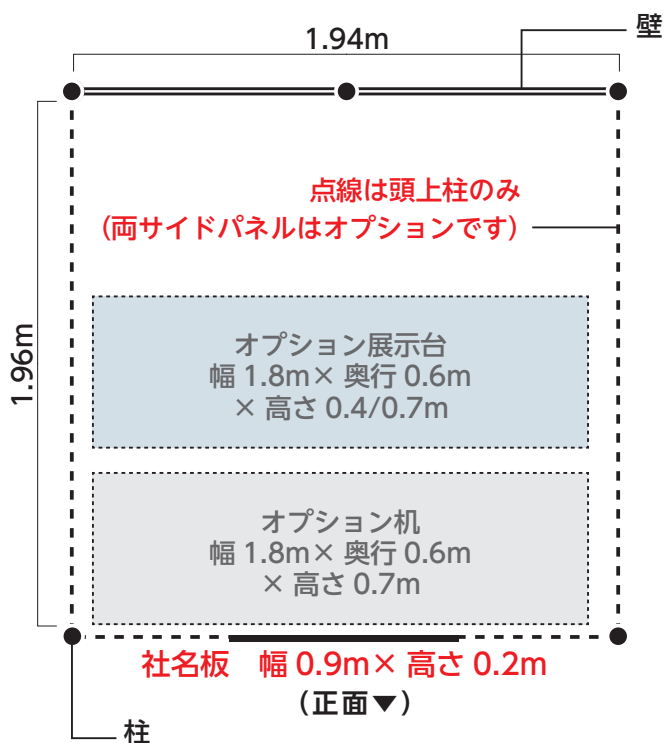
【基礎小間（1小間）平面図】
